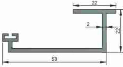
3668 0,563 kg/m
