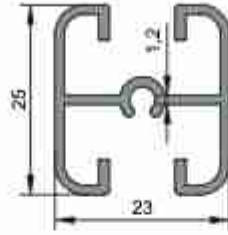
1742 0,360 kg/m
