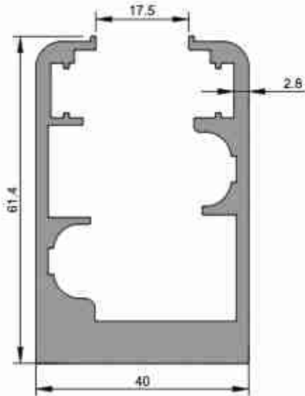
2574 Küpeşte Profil 1,480 kg/m
