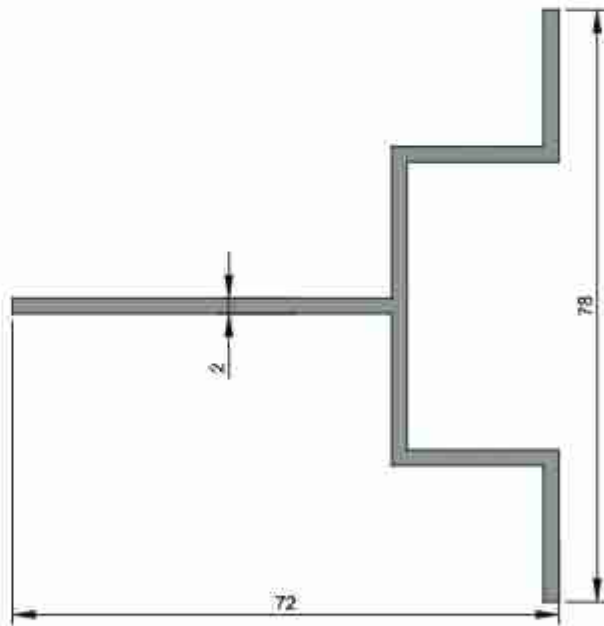
3192 0,910 kg/m
