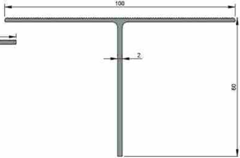
1797 0,742 kg/m
