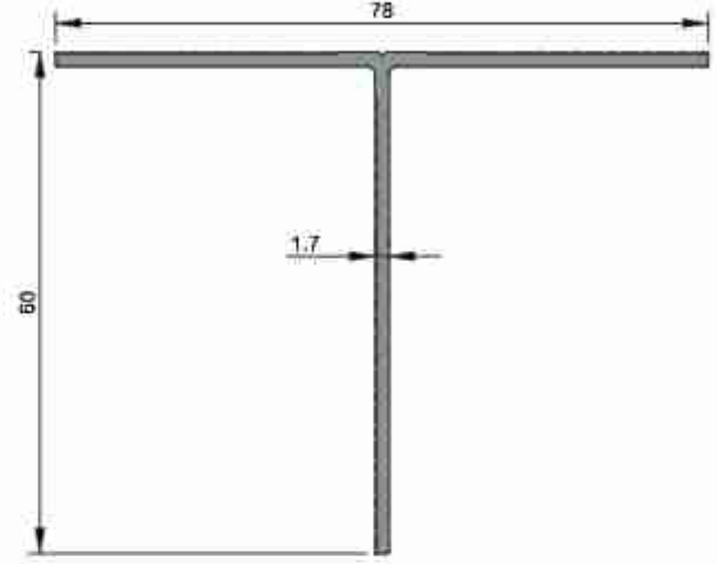
1170 0,578 kg/m
