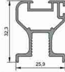
1530 0,549 kg/m
