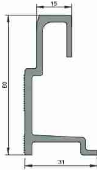
2634 0,909 kg/m
