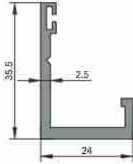
4015 0,461 kg/m
