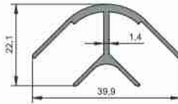
1291 0,311 kg/m
