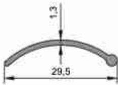
1708 0,118 kg/m
