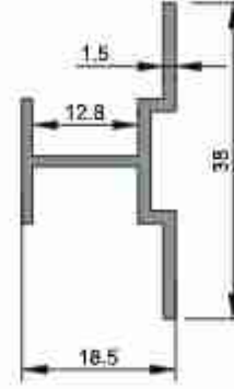
3777 0,269 kg/m
