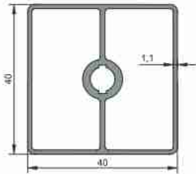
1245 0,695 kg/m
