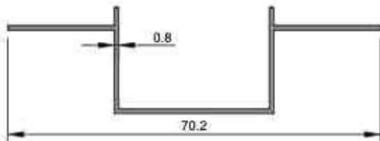
1832 0,235 kg/m
