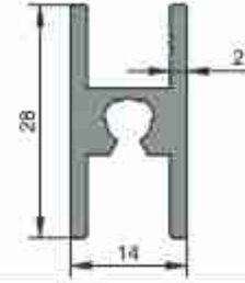
1666 0,434 kg/m
