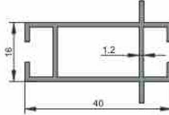
1246 0,727 kg/m
