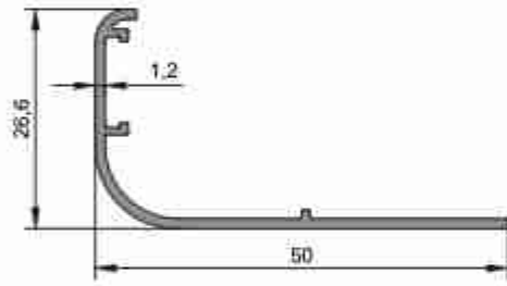
1713 0,259 kg/m
