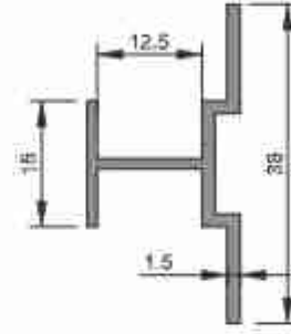
3221 0,268 kg/m
