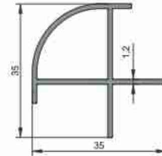
1814 0,356 kg/m
