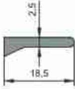
1712 0,141 kg/m
