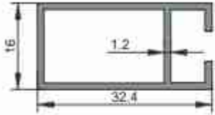
1399 0,540 kg/m
