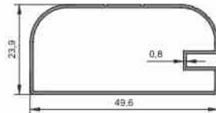
1309 0,326 kg/m
