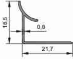
1574 0,101 kg/m
