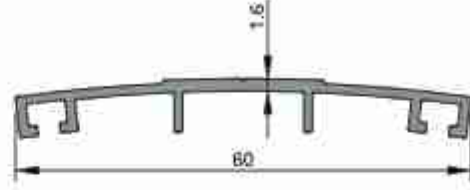
1756 0,319 kg/m
