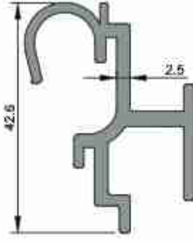
1754 0,718 kg/m
