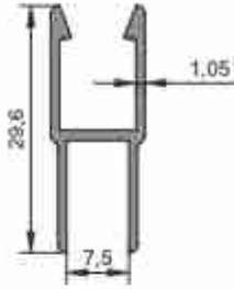
1620 0,209 kg/m
