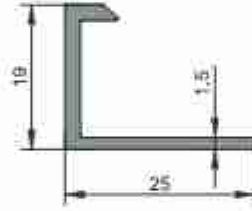
1377 0,218 kg/m
