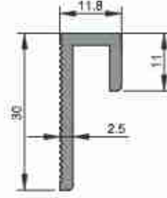
2901 0,297 kg/m
