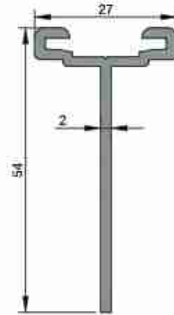
1394 0,479 kg/m
