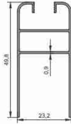
2047 0,385 kg/m
