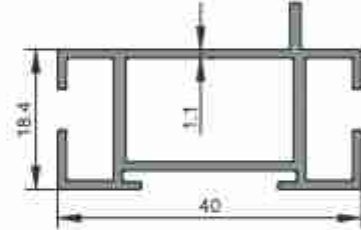
1802 0,768kg/m
