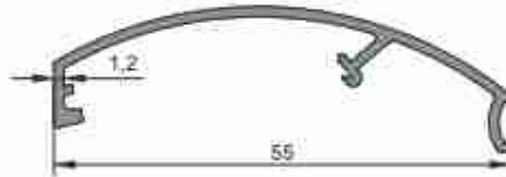
1460 0,279 kg/m
