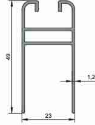
1743 0,506 kg/m
