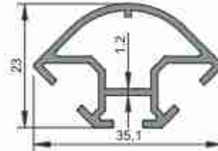
1051 0,606 kg/m
