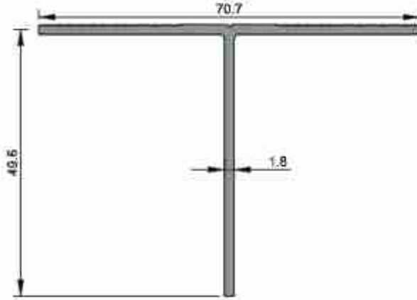
1158 0,560 kg/m
