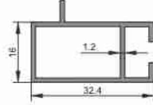
1061 0,572 kg/m
