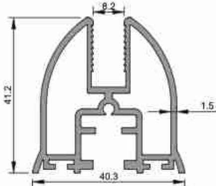
2576 Küpeşte Profil 0,921 kg/m
