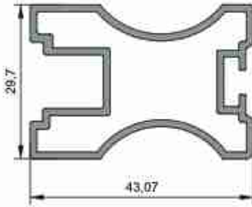
1638 0,676 kg/m
