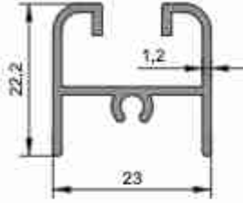
1741 0,294 kg/m
