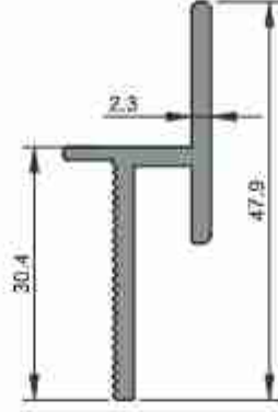
3955 0,436 kg/m
