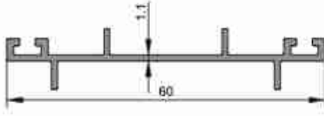
1755 0,290 kg/m
