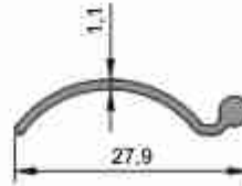
1710 0,112 kg/m
