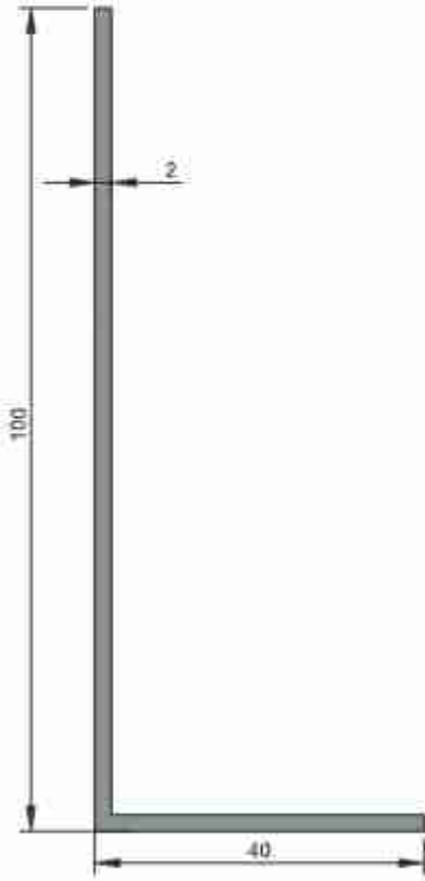
3748 0,748 kg/m
