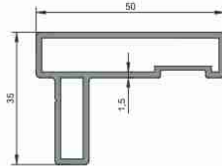
1293 0,883 kg/m
