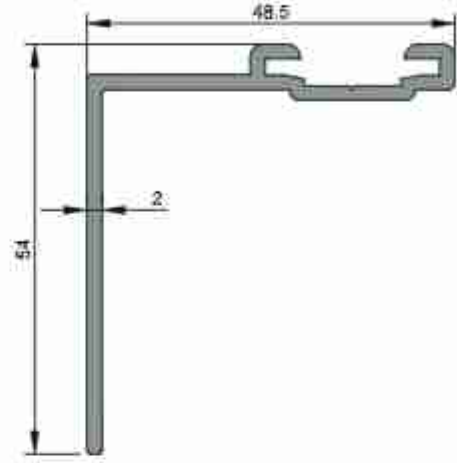
1255 0,603 kg/m
