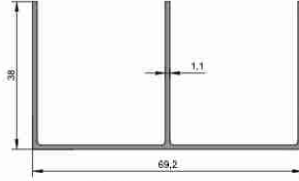
1608 0,538 kg/m
