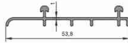
1547 0,236 kg/m
