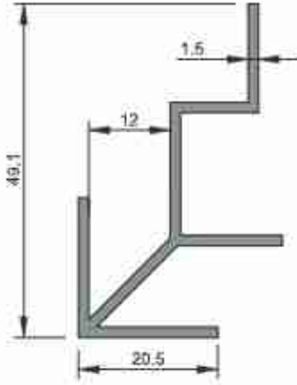
3220 0,484 kg/m
