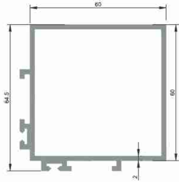
3026 1,531 kg/m
