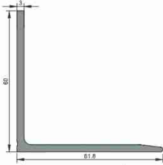
2637 0,954 kg/m
